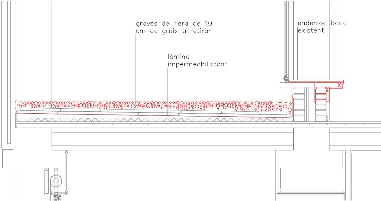
Secció tipus enderrocs e:1/25
