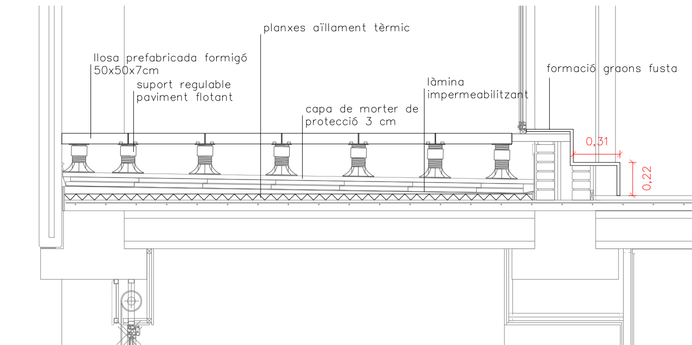
Secció tipus e:1/25
